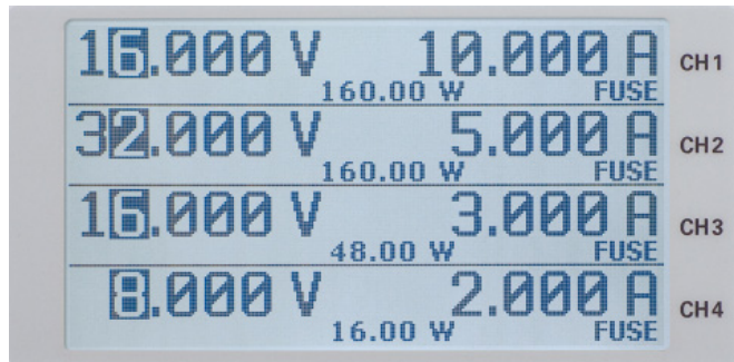
Fig. 5.1: Position 1V pour les 4 voies
