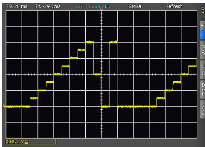
Fig. 3.3: Fonction arbitraire en escalier
