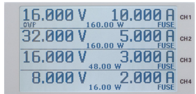
Fig. 5.6: OVP (Protection contre les surtensions)
