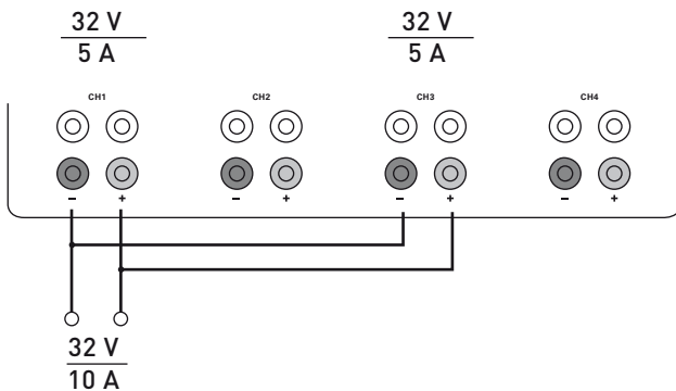
Fig. 7.2: Exemple de fonctionnement en série
