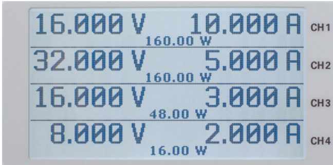
Fig. 4.1: Réglage des valeurs maximales pour HMP4040
