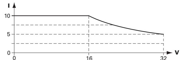
Fig. 4.4: HMP4030/40 L'hyperbole de puissance
