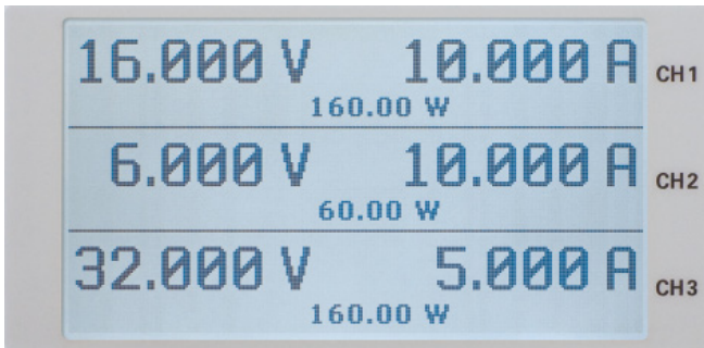
Fig. 4.2: Réglage des valeurs maximales pour HMP4030
