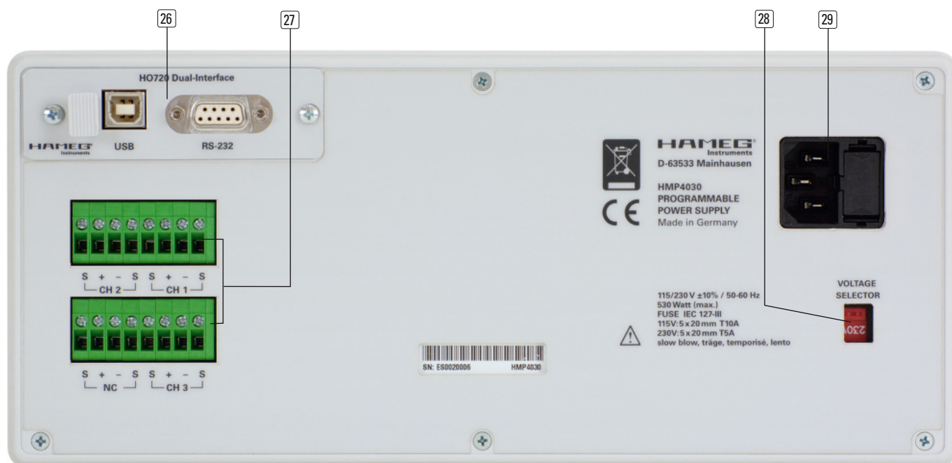
Fig. 2.2: Face arrière de HMP4030 / HMP4040
