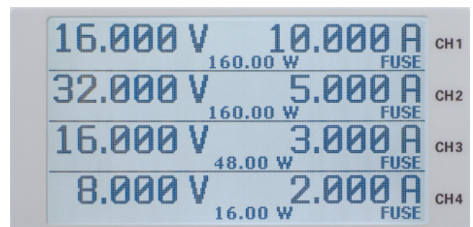
Fig. 4.5: Fusible électronique activé - affichage à l'écran
