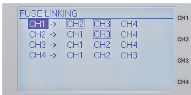
Fig. 3.2: Fonction Fuse Linking activée (écran de présentation)
