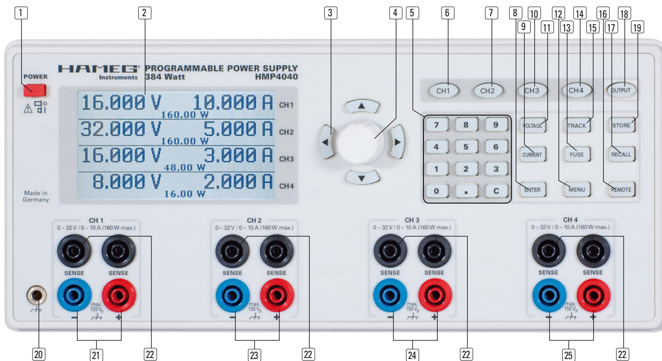
Fig. 2.1: Face avant de HMP4040
